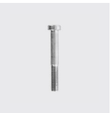
DIN 7984 Vis à tête cylindrique à six pans creux, à tête basse DIN 7984 Matériau: A4, Type de matériau: acier inoxydable, Longueur mm: 35, Filetage: M8, ID unique: D7984+8x35, SKU 5147408035
