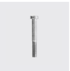
DIN 7984 Vis à tête cylindrique à six pans creux, à tête basse DIN 7984 Longueur mm: 25, Filetage: M5, Type de matériau: acier inoxydable, ID unique: D7984-5x25, Matériau: A2, SKU 5147205025
