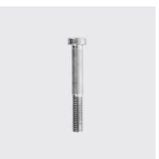
DIN 7984 Vis à tête cylindrique à six pans creux, à tête basse DIN 7984 Filetage: M5, ID unique: D7984-5x40, Type de matériau: acier inoxydable, Matériau: A2, Longueur mm: 40, SKU 5147205040
