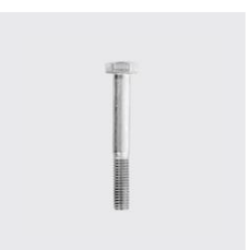
DIN 931 Vis à tête six pans, partiellement filetée DIN 931 Filetage: M6, Type de matériau: acier inoxydable, Longueur mm: 40, Matériau: A4, ID unique: D931+6x40, SKU 5112406040
