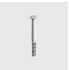
DIN 931 Vis à tête six pans, partiellement filetée DIN 931 Filetage: M5, Type de matériau: acier inoxydable, Matériau: A4, Longueur mm: 55, ID unique: D931+5x55, SKU 5112405055
