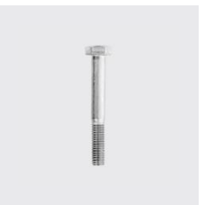
DIN 931 Vis à tête six pans, partiellement filetée DIN 931 Filetage: M5, Type de matériau: acier inoxydable, Longueur mm: 40, ID unique: D931+5x40, Matériau: A4, SKU 5112405040
