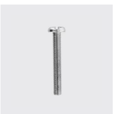
DIN 85 A Vis à tête aplatie Pan Head avec fente DIN 85 A Type de matériau: acier inoxydable, Matériau: A2, ID unique: D85-6x45, Longueur mm: 45, Filetage: M6, SKU 5122206045
