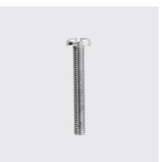
DIN 85 A Vis à tête aplatie Pan Head avec fente DIN 85 A Filetage: M3, Type de matériau: acier inoxydable, Matériau: A2, Longueur mm: 25, ID unique: D85-3x25, SKU 5122203025
