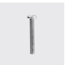
DIN 85 A Vis à tête aplatie Pan Head avec fente DIN 85 A Filetage: M3, Type de matériau: acier inoxydable, Matériau: A2, Longueur mm: 16, ID unique: D85-3x16, SKU 5122203016
