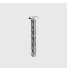
DIN 85 A Vis à tête aplatie Pan Head avec fente DIN 85 A Filetage: M3, Type de matériau: acier inoxydable, Matériau: A2, Longueur mm: 30, ID unique: D85-3x30, SKU 5122203030
