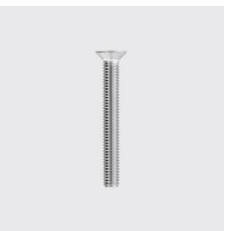
DIN 965 A Senkschraube mit Kreuzschlitz Phillips Form H DIN 965 A Materialart: Edelstahl rostbeständig, Gewinde: M3, Länge mm: 6, Unique-Id: D965-3x6, Werkstoff: A2, SKU 5131203006
