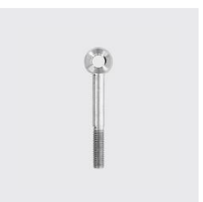
DIN 444 B Vis à oeillet forme B, surfaces planes tra- vallées DIN 444 Longueur mm: 120, ID unique: D444-20x120, Type de matériau: acier inoxydable, Filetage: M20, Matériau: A2, SKU 5235220120
