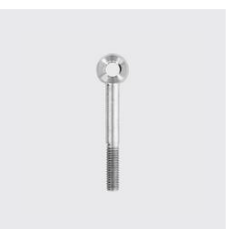
DIN 444 B Vis à oeillet forme B, surfaces planes tra- vallées DIN 444 Type de matériau: acier inoxydable, Longueur mm: 140, Filetage: M20, Matériau: A2, ID unique: D444-20x140, SKU 5235220140
