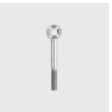
DIN 444 B Vis à oeillet forme B, surfaces planes tra- vallées DIN 444 Longueur mm: 100, Type de matériau: acier inoxydable, ID unique: D444-12x100, Filetage: M12, Matériau: A2, SKU 5235212100
