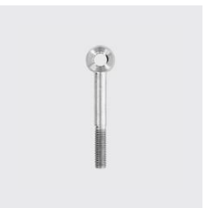
DIN 444 B Vis à oeillet forme B, surfaces planes tra- vallées DIN 444 Longueur mm: 120, ID unique: D444-12x120, Type de matériau: acier inoxydable, Filetage: M12, Matériau: A2, SKU 5235212120
