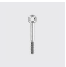
DIN 444 B Vis à oeillet forme B, surfaces planes tra- vallées DIN 444 Filetage: M16, Type de matériau: acier inoxydable, Longueur mm: 60, ID unique: D444-16x60, Matériau: A2, SKU 5235216060
