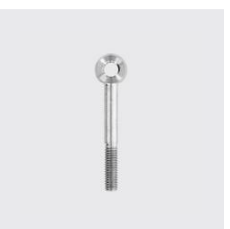
DIN 444 B Vis à oeillet forme B, surfaces planes tra- vallées DIN 444 Longueur mm: 80, Type de matériau: acier inoxydable, Filetage: M20, ID unique: D444-20x80, Matériau: A2, SKU 5235220080
