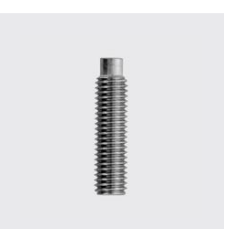
DIN 915 Vis sans tête à six pans creux, à téton ISO 4028 (ex. DIN 915) Longueur mm: 25, Type de matériau: acier inoxydable, ID unique: D915-8x25, Matériau: A2, Filetage: M8, SKU 5143208025
