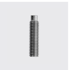
DIN 915 Vis sans tête à six pans creux, à téton ISO 4028 (ex. DIN 915) Type de matériau: acier inoxydable, Matériau: A2, Filetage: M6, Longueur mm: 40, ID unique: D915-6x40, SKU 5143206040
