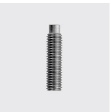
DIN 915 Vis sans tête à six pans creux, à téton ISO 4028 (ex. DIN 915) Type de matériau: acier inoxydable, Matériau: A2, Filetage: M8, Longueur mm: 12, ID unique: D915-8x12, SKU 5143208012
