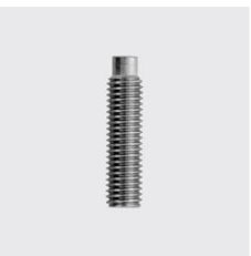
DIN 915 Vis sans tête à six pans creux, à téton ISO 4028 (ex. DIN 915) Longueur mm: 16, Type de matériau: acier inoxydable, ID unique: D915-8x16, Matériau: A2, Filetage: M8, SKU 5143208016
