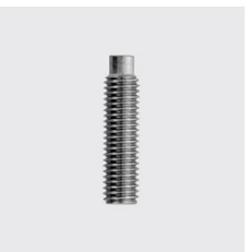
DIN 915 Vis sans tête à six pans creux, à téton ISO 4028 (ex. DIN 915) Type de matériau: acier inoxydable, Matériau: A2, Filetage: M6, Longueur mm: 35, ID unique: D915-6x35, SKU 5143206035
