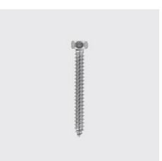
DIN 7976 C Sechskant-Blechschraube mit Spitze Form C DIN 7976 C Unique-Id: D7976C-5-5x19, Materialart: Edelstahl rost- beständig, Länge mm: 19, Ausssen-Ø mm: 5,5, Werkstoff: A2, SKU 5167255019
