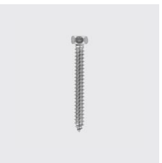
DIN 7976 C Sechskant-Blechschraube mit Spitze Form C DIN 7976 C Unique-Id: D7976C-4-2x25, Materialart: Edelstahl rost- beständig, Werkstoff: A2, Länge mm: 25, Ausssen-Ø mm: 4,2, SKU 5167242025
