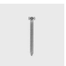
DIN 7976 C Sechskant-Blechschraube mit Spitze Form C DIN 7976 C Länge mm: 45, Materialart: Edelstahl rostbeständig, Ausssen-Ø mm: 4,8, Unique-Id: D7976C-4-8x45, Werk- stoff: A2, SKU 5167248045
