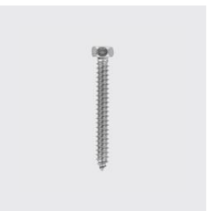
DIN 7976 C Sechskant-Blechschraube mit Spitze Form C DIN 7976 C Materialart: Edelstahl rostbeständig, Ausssen-Ø mm: 4,8, Unique-Id: D7976C-4-8x38, Werkstoff: A2, Länge mm: 38, SKU 5167248038
