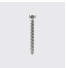
DIN 7976 C Sechskant-Blechschraube mit Spitze Form C DIN 7976 C Materialart: Edelstahl rostbeständig, Werkstoff: A2, Länge mm: 38, Unique-Id: D7976C-6-3x38, Ausssen-Ø mm: 6,3, SKU 5167263038
