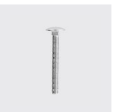
DIN 603 Vis à tête bombée avec collet carré, sans écrou six pans DIN 603 Filetage: M6, Matériau: A2, Type de matériau: acier inoxydable, ID unique: D603-6x20, Longueur mm: 20, SKU 5134206020
