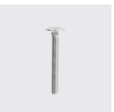
DIN 603 Vis à tête bombée avec collet carré, sans écrou six pans DIN 603 Filetage: M5, Longueur mm: 50, Matériau: A2, Type de matériau: acier inoxydable, ID unique: D603-5x50, SKU 5134205050
