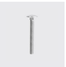
DIN 603 Vis à tête bombée avec collet carré, sans écrou six pans DIN 603 Filetage: M5, Matériau: A2, Longueur mm: 25, Type de matériau: acier inoxydable, ID unique: D603-5x25, SKU 5134205025
