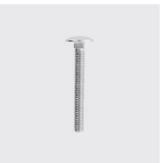
DIN 603 Vis à tête bombée avec collet carré, sans écrou six pans DIN 603 Filetage: M5, Matériau: A2, Longueur mm: 30, Type de matériau: acier inoxydable, ID unique: D603-5x30, SKU 5134205030
