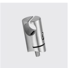
GN-6522 Halter für Einfassprofil, geschliffen, inkl. Montageschraube für Rohr mm: flach/plat, Materialart: Edelstahl rostbeständig, Unique-Id: GN6522 flach, Werkstoff: 304, SKU 188735030
