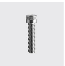
K-210 Vis à tête cylindrique à six pans creux, à filetage UNC Matériau: A4, ID unique: K210+3/8x51, Longueur mm: 51, Type de matériau: acier inoxydable, Filetage POUCE : 3/8, SKU 514943051
