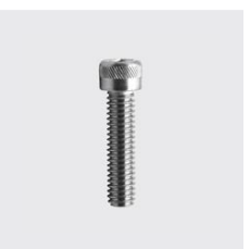
K-210 Vis à tête cylindrique à six pans creux, à filetage UNC Longueur mm: 38, Matériau: A4, Filetage POUCE : 5/8, ID unique: K210+5/8x38, Type de matériau: acier inoxydable, SKU 514945038
