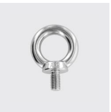
K-265 Ringschraube, gegossen, Form nach DIN 580 Werkstoff: A4, Materialart: Edelstahl rostbeständig, Gewinde: M20, Unique-Id: K265+20, SKU 5247420
