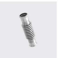
P-741 Compensateur d'expansion PN10, inox-PRES® Type de matériau: acier inoxydable, Matériau: 1.4404, Ø extérieur mm: 54, Longueur mm: 221, ID unique: P741 54, SKU 14150540
