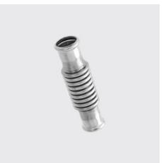
P-741 Compensateur d'expansion PN10, inox-PRES® Type de matériau: acier inoxydable, Matériau: 1.4404, ID unique: P741 22, Longueur mm: 139, Ø extérieur mm: 22, SKU 14150220
