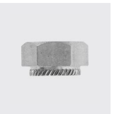
K-297 Einpressmutter Materialart: Edelstahl rostbeständig, Unique-Id: K297-5, Werkstoff: A1, Gewinde: M5, SKU 5218205
