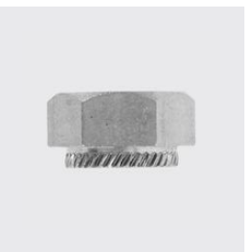
K-297 Einpressmutter Materialart: Edelstahl rostbeständig, Gewinde: M4, Unique-Id: K297-4, Werkstoff: A1, SKU 5218204
