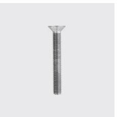
DIN 7991 Senkschraube mit Innensechskant, Ganzgewinde ISO 10642, vormals (DIN 7991) Materialart: Edelstahl rostbeständig, Länge mm: 70, Gewinde: M12, Werkstoff: A4, Unique-Id: D7991+12x70, SKU 5145412070
