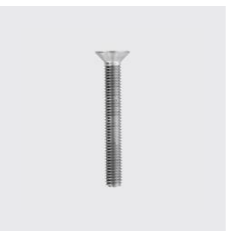
DIN 7991 Senkschraube mit Innensechskant, Ganzgewinde ISO 10642, vormals (DIN 7991) Materialart: Edelstahl rostbeständig, Länge mm: 80, Gewinde: M12, Unique-Id: D7991+12x80, Werkstoff: A4, SKU 5145412080
