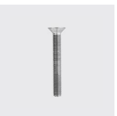
DIN 7991 Senkschraube mit Innensechskant, Ganzgewinde ISO 10642, vormals (DIN 7991) Unique-Id: D7991+16x30, Materialart: Edelstahl rostbeständig, Gewinde: M16, Länge mm: 30, Werkstoff: A4, SKU 5145416030
