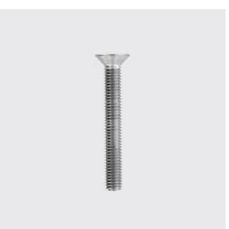
DIN 7991 Senkschraube mit Innensechskant, Ganzgewinde ISO 10642, vormals (DIN 7991) Materialart: Edelstahl rostbeständig, Länge mm: 35, Gewinde: M16, Unique-Id: D7991+16x35, Werkstoff: A4, SKU 5145416035
