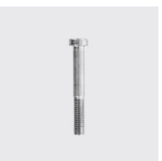
DIN 7984 Vis à tête cylindrique à six pans creux, à tête basse DIN 7984 Filetage: M10, Matériau: A4, ID unique: D7984+10X20, Type de matériau: acier inoxydable, Longueur mm: 20, SKU 5147410020
