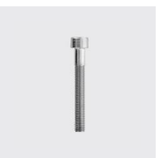
DIN 912 Zylinderschraube mit Innensechskant, mit Schaft DIN 912 Unique-Id: D912-12x180, Werkstoff: A2, Gewinde: M12, Länge mm: 180, Materialart: Edelstahl rostbeständig, SKU 5140212180
