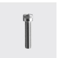
K-210 Vis à tête cylindrique à six pans creux, à filetage UNC Matériau: A4, ID unique: K210+3/8x25, Type de matériau: acier inoxydable, Longueur mm: 25, Filetage POUCE : 3/8, SKU 514943025
