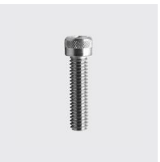
K-210 Vis à tête cylindrique à six pans creux, à filetage UNC Matériau: A4, Filetage POUCE : 5/16, Longueur mm: 32, Type de matériau: acier inoxydable, ID unique: K210+5/16x32, SKU 514942032
