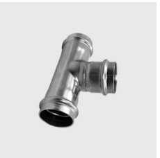
PU-760 Té égal, inoxPRES UNIKO® Type de matériau: acier inoxydable, Ø extérieur mm: 28, Matériau: 1.4404, ID unique: PU760 28, SKU 141270615
