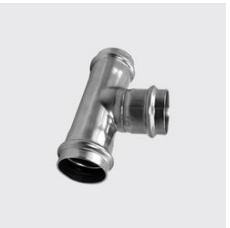
PU-760 Té égal, inoxPRES UNIKO® Type de matériau: acier inoxydable, ID unique: PU760 35, Matériau: 1.4404, Ø extérieur mm: 35, SKU 141270620
