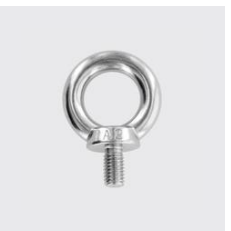
K-265 Ringschraube, gegossen, Form nach DIN 580 Gewinde: M8, Werkstoff: A4, Materialart: Edelstahl rostbeständig, Unique-Id: K265+8, SKU 5247408
