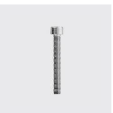
DIN 912 Vis à tête cylindrique à six pans creux, entièrement filetée DIN 912 Longueur mm: 20, Filetage: M12, Type de matériau: acier inoxydable, ID unique: D912+12x20, Matériau: A4, SKU 5140412020
