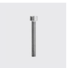
DIN 912 Vis à tête cylindrique à six pans creux, entièrement filetée DIN 912 Filetage: M10, Type de matériau: acier inoxydable, Longueur mm: 35, Matériau: A4, ID unique: D912+10x35, SKU 5140410035
