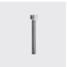
DIN 912 Vis à tête cylindrique à six pans creux, entièrement filetée DIN 912 Longueur mm: 25, Filetage: M6, Type de matériau: acier inoxydable, ID unique: D912+6x25, Matériau: A4, SKU 5140406025
