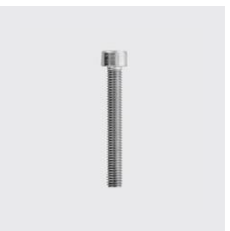
DIN 912 Vis à tête cylindrique à six pans creux, entièrement filetée DIN 912 Longueur mm: 25, Filetage: M10, ID unique: D912-10x25, Type de matériau: acier inoxydable, Matériau: A2, SKU 5140210025
