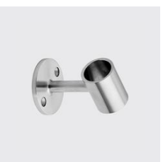
GB-3174 Rohrhater, geschliffen Materialart: Edelstahl rostbeständig, Loch-Ø mm: 6, für Rohr mm: 48.3, Rondellen-Ø mm: 70, Werkstoff: 316, Unique-Id: GB3174 48.3, SKU 188702650
