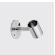
GB-3174 Rohrhater, geschliffen Materialart: Edelstahl rostbeständig, für Rohr mm: 42.4, Unique-Id: GB3174 42.4, Loch-Ø mm: 6, Rondellen-Ø mm: 70, Werkstoff: 316, SKU 188702640
