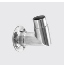
GB-3164 Flanschbohrer 90°, geschliffen für Rohr mm: 42.4, Materialart: Edelstahl rostbeständig, Werkstoff: 316, Unique-Id: GB3164 42.4, SKU 188702044
