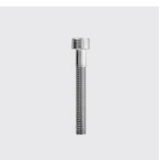
DIN 912 Vis à tête cylindrique à six pans creux, par-tiellement filetée DIN 912 Filetage: M16, Matériau: A4, ID unique: D912+16x75, Type de matériau: acier inoxydable, Longueur mm: 75, SKU 5140416075
