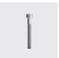
DIN 912 Vis à tête cylindrique à six pans creux, par-tiellement filetée DIN 912 Matériau: A4, Longueur mm: 60, ID unique: D912+10x60, Type de matériau: acier inoxydable, Filetage: M10, SKU 5140410060
