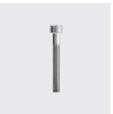
DIN 912 Vis à tête cylindrique à six pans creux, par-tiellement filetée DIN 912 Matériau: A4, Type de matériau: acier inoxydable, ID unique: D912+10x130, Filetage: M10, Longueur mm: 130, SKU 5140410130
