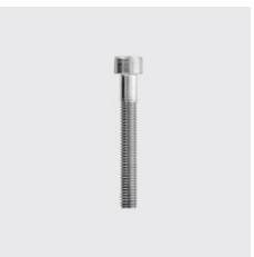
DIN 912 Vis à tête cylindrique à six pans creux, par-tiellement filetée DIN 912 Matériau: A2, Longueur mm: 110, Filetage: M24, ID unique: D912-24x110, Type de matériau: acier inoxydable, SKU 5140224110
