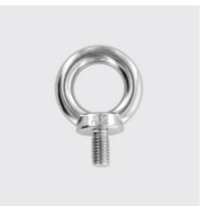
K-265 Vis à anneau, pièce coulée, forme selon DIN 580 Filetage: M8, Matériau: A4, Type de matériau: acier inoxydable, ID unique: K265+8, SKU 5247408
