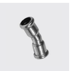
P-706 Bogen 15° , innen - innen, inoxPRES® Unique-Id: P706 88.9, Materialart: Edelstahl rost- beständig, Aussen-Ø mm: 88.9, Werkstoff: 1.4404, SKU 141141070
