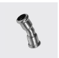
P-706 Bogen 15° , innen - innen, inoxPRES® Unique-Id: P706 108, Aussen-Ø mm: 108, Materi- alart: Edelstahl rostbeständig, Werkstoff: 1.4404, SKU 141141080
