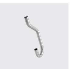
P-718 Sprungbogen 180° , inoxPRES® Unique-id: P718 28, Materialart: Edelstahl rostbeständig, Werkstoff: 1.4404, Ausssen-Ø mm: 28, SKU 141186280
