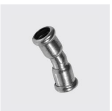
P-706 Bogen 15° , innen - innen, inoxPRES® Unique-Id: P706 18, Aussen-Ø mm: 18, Materialart: Edelstahl rostbeständig, Werkstoff: 1.4404, SKU 141141005
