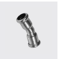
P-706 Bogen 15° , innen - innen, inoxPRES® Aussen-Ø mm: 22, Unique-Id: P706 22, Materi- alart: Edelstahl rostbeständig, Werkstoff: 1.4404, SKU 141141010
