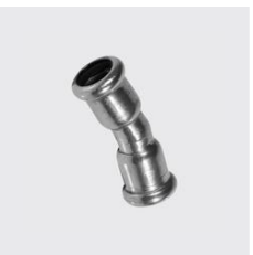
P-706 Bogen 15° , innen - innen, inoxPRES® Aussen-Ø mm: 42, Unique-Id: P706 42, Materi- alart: Edelstahl rostbeständig, Werkstoff: 1.4404, SKU 141141040
