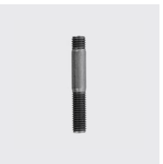
DIN 939 Stiftschraube Einschraubende 1,25 d DIN 939 Materialart: Edelstahl rostbeständig, Länge mm: 35, Gewinde: M10, Unique-Id: D939+10x35, Werkstoff: A4, SKU 5234410035
