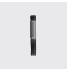
DIN 939 Stiftschraube Einschraubende 1,25 d DIN 939 Materialart: Edelstahl rostbeständig, Werkstoff: A2, Länge mm: 80, Gewinde: M6, Unique-Id: D939-6X80, SKU 5234206080
