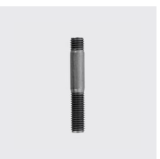
DIN 939 Stiftschraube Einschraubende 1,25 d DIN 939 Materialart: Edelstahl rostbeständig, Unique-Id: D939+12x55, Gewinde: M12, Werkstoff: A4, Länge mm: 55, SKU 5234412055
