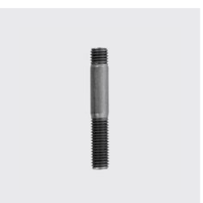
DIN 939 Stiftschraube Einschraubende 1,25 d DIN 939 Materialart: Edelstahl rostbeständig, Länge mm: 100, Werkstoff: A2, Unique-Id: D939-16x100, Gewinde: M16, SKU 5234216100
