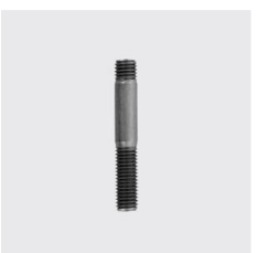
DIN 939 Stiftschraube Einschraubende 1,25 d DIN 939 Materialart: Edelstahl rostbeständig, Unique-Id: D939+16x70, Gewinde: M16, Werkstoff: A4, Länge mm: 70, SKU 5234416070
