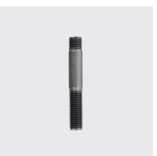
DIN 939 Stiftschraube Einschraubende 1,25 d DIN 939 Materialart: Edelstahl rostbeständig, Länge mm: 60, Unique-Id: D939+10x60, Gewinde: M10, Werkstoff: A4, SKU 5234410060
