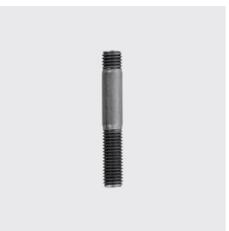
DIN 939 Stiftschraube Einschraubende 1,25 d DIN 939 Materialart: Edelstahl rostbeständig, Länge mm: 40, Gewinde: M10, Unique-Id: D939+10x40, Werkstoff: A4, SKU 5234410040
