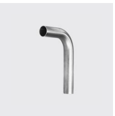
P-711 Tuyau cintré 90°, inoxPRES® Ø extérieur mm: 28, ID unique: P711 28, Type de matéri- au: acier inoxydable, Matériau: 1.4404, SKU 14119280
