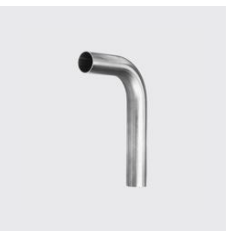
P-711 Tuyau cintré 90°, inoxPRES® Ø extérieur mm: 35, ID unique: P711 35, Type de matéri- au: acier inoxydable, Matériau: 1.4404, SKU 14119350
