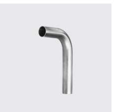
P-711 Tuyau cintré 90°, inoxPRES® Ø extérieur mm: 76.1, ID unique: P711 76.1 E, Type de matériau: acier inoxydable, Matériau: 1.4404, SKU 141197600
