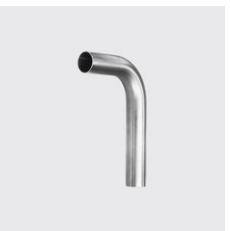
P-711 Tuyau cintré 90°, inoxPRES® ID unique: P711 22, Type de matériau: acier inoxydable, Matériau: 1.4404, Ø extérieur mm: 22, SKU 14119220
