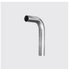
P-711 Tuyau cintré 90°, inoxPRES® Ø extérieur mm: 54, ID unique: P711 54, Type de matéri- au: acier inoxydable, Matériau: 1.4404, SKU 14119540
