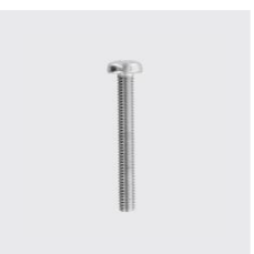
DIN 7985 A Vis à tête bombée à empreinte cruciforme H (Phillips) DIN 7985 A ID unique: D7985-3x30, Filetage: M3, Matériau: A2, Type de matériau: acier inoxydable, Longueur mm: 30, SKU 5133203030
