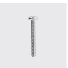
DIN 7985 A Vis à tête bombée à empreinte cruciforme H (Phillips) DIN 7985 A Matériau: A2, ID unique: D7985-8x35, Type de matériau: acier inoxydable, Filetage: M8, Longueur mm: 35, SKU 5133208035
