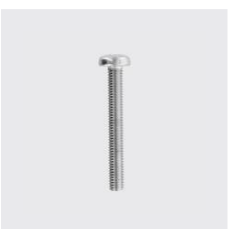
DIN 7985 A Vis à tête bombée à empreinte cruciforme H (Phillips) DIN 7985 A Filetage: M3, Matériau: A2, Type de matériau: acier inoxydable, Longueur mm: 35, ID unique: D7985-3x35, SKU 5133203035
