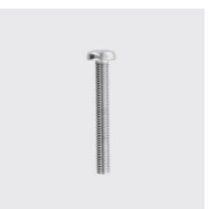
DIN 7985 A Vis à tête bombée à empreinte cruciforme H (Phillips) DIN 7985 A Longueur mm: 16, Filetage: M3, Matériau: A2, Type de matériau: acier inoxydable, ID unique: D7985-3x16, SKU 5133203016
