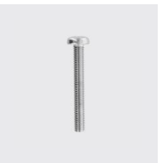
DIN 7985 A Vis à tête bombée à empreinte cruciforme H (Phillips) DIN 7985 A Matériau: A2, Type de matériau: acier inoxydable, Longueur mm: 80, ID unique: D7985-6x80, Filetage: M6, SKU 5133206080
