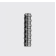
DIN 913 Gewindestift mit Innensechskant und Kegekuppe ISO 4026 formals (DIN 913) Gewinde: M12, Materialart: Edelstahl rostbeständig, Werkstoff: A2, Länge mm: 12, Unique-Id: D913-12x12, SKU 5141212012
