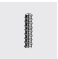
DIN 913 Gewindestift mit Innensechskant und Kegekuppe ISO 4026 vormals (DIN 913) Länge mm: 8, Werkstoff: A4, Materialart: Edelstahl rostbeständig, Gewinde: M5, Unique-Id: D913+5x8, SKU 5141405008
