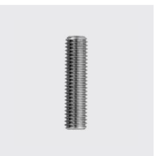
DIN 913 Gewindestift mit Innensechskant und Kegelekuppe ISO 4026 vormals (DIN 913) Materialart: Edelstahl rostbeständig, Unique-Id: D913-5x6, Gewinde: M5, Länge mm: 6, Werkstoff: A2, SKU 5141205006
