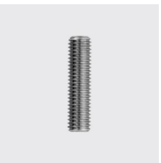
DIN 913 Gewindestift mit Innensechskant und Kegelekuppe ISO 4026 vormals (DIN 913) Unique-Id: D913-10x25, Werkstoff: A4, Materialart: Edelstahl rostbeständig, Länge mm: 25, Gewinde: M10, SKU 5141410025
