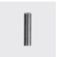
DIN 913 Gewindestift mit Innensechskant und Kegelekuppe ISO 4026 vormals (DIN 913) Unique-Id: D913-12x35, Gewinde: M12, Materialart: Edelstahl rostbeständig, Werkstoff: A2, Länge mm: 35, SKU 5141212035
