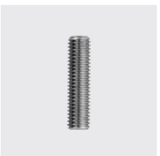
DIN 913 Gewindestift mit Innensechskant und Kegelekuppe ISO 4026 vormals (DIN 913) Länge mm: 16, Materialart: Edelstahl rostbeständig, Gewinde: M3, Werkstoff: A2, Unique-Id: D913-3x16, SKU 5141203016
