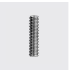
DIN 913 Gewindestift mit Innensechskant und Kegekuppe ISO 4026 formals (DIN 913) Materialart: Edelstahl rostbeständig, Länge mm: 45, Unique-Id: D913-6x45, Werkstoff: A2, Gewinde: M6, SKU 5141206045
