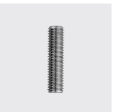
DIN 913 Gewindestift mit Innensechskant und Kegelekuppe ISO 4026 vormals (DIN 913) Materialart: Edelstahl rostbeständig, Unique-Id: D913-6x35, Werkstoff: A2, Länge mm: 35, Gewinde: M6, SKU 5141206035
