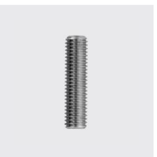
DIN 913 Gewindestift mit Innensechskant und Kegekuppe ISO 4026 vormals (DIN 913) Werkstoff: A4, Materialart: Edelstahl rostbeständig, Gewinde: M5, Unique-Id: D913+5x5, Länge mm: 5, SKU 5141405005
