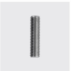
DIN 913 Gewindestift mit Innensechskant und Kegelekuppe ISO 4026 vormals (DIN 913) Länge mm: 16, Werkstoff: A4, Materialart: Edelstahl rostbeständig, Unique-Id: D913+6x16, Gewinde: M6, SKU 5141406016
