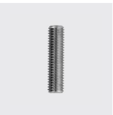
DIN 913 Gewindestift mit Innensechskant und Kegelekuppe ISO 4026 vormals (DIN 913) Länge mm: 16, Gewinde: M4, Materialart: Edelstahl rostbeständig, Werkstoff: A2, Unique-Id: D913-4x16, SKU 5141204016
