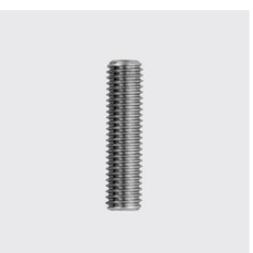
DIN 913 Gewindestift mit Innensechskant und Kegekuppe ISO 4026 formals (DIN 913) Materialart: Edelstahl rostbeständig, Länge mm: 30, Gewinde: M10, Unique-Id: D913-10x30, Werkstoff: A2, SKU 5141210030
