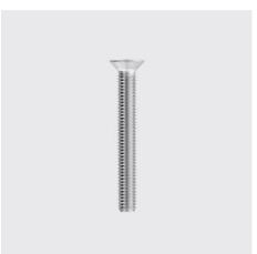
DIN 965 A Senkschraube mit Kreuzschlitz Phillips Form H DIN 965 A Länge mm: 8, Materialart: Edelstahl rostbeständig, Gewinde: M3, Unique-Id: D965-3x8, Werkstoff: A2, SKU 5131203008
