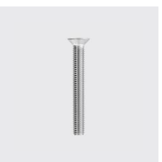
DIN 965 A Senkschraube mit Kreuzschlitz Phillips Form H DIN 965 A Materialart: Edelstahl rostbeständig, Länge mm: 30, Unique-Id: D965-3x30, Gewinde: M3, Werkstoff: A2, SKU 5131203030
