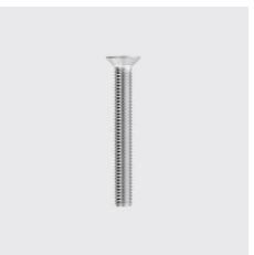
DIN 965 A Senkschraube mit Kreuzschlitz Phillips Form H DIN 965 A Materialart: Edelstahl rostbeständig, Länge mm: 40, Unique-Id: D965-5x40, Gewinde: M5, Werkstoff: A2, SKU 5131205040
