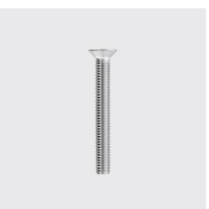
DIN 965 A Senkschraube mit Kreuzschlitz Phillips Form H DIN 965 A Materialart: Edelstahl rostbeständig, Länge mm: 45, Unique-Id: D965-5x45, Gewinde: M5, Werkstoff: A2, SKU 5131205045
