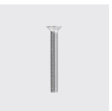
DIN 965 A Senkschraube mit Kreuzschlitz Phillips Form H DIN 965 A Materialart: Edelstahl rostbeständig, Gewinde: M6, Länge mm: 100, Unique-Id: D965-6x100, Werkstoff: A2, SKU 5131206100
