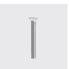
DIN 965 A Senkschraube mit Kreuzschlitz Phillips Form H DIN 965 A Länge mm: 50, Materialart: Edelstahl rostbeständig, Unique-Id: D965-10x50, Werkstoff: A2, Gewinde: M10, SKU 5131210050
