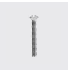
DIN 964 A Vis à tête fraisée bombée avec fente DIN 964 A Filetage: M5, Type de matériau: acier inoxydable, Longueur mm: 80, ID unique: D964-5x80, Matériau: A2, SKU 5124205080
