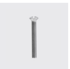
DIN 964 A Vis à tête fraisée bombée avec fente DIN 964 A Type de matériau: acier inoxydable, Longueur mm: 10, Filetage: M6, Matériau: A2, ID unique: D964-6x10, SKU 5124206010
