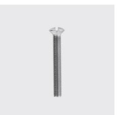
DIN 964 A Vis à tête fraisée bombée avec fente DIN 964 A Type de matériau: acier inoxydable, Filetage: M6, Matériau: A2, ID unique: D964-6x16, Longueur mm: 16, SKU 5124206016
