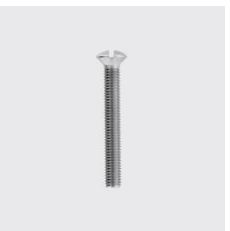
DIN 964 A Vis à tête fraisée bombée avec fente DIN 964 A Filetage: M5, Type de matériau: acier inoxydable, Longueur mm: 70, Matériau: A2, ID unique: D964-5x70, SKU 5124205070
