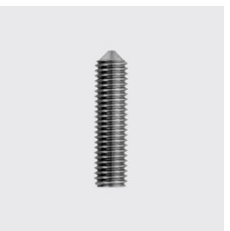
DIN 914 Vis sans tête à six pans creux, bout pointu ISO 4027 (ex. DIN 914) Longueur mm: 40, ID unique: D914-10x40, Matériau: A2, Filetage: M10, Type de matériau: acier inoxydable, SKU 5142210040
