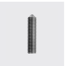
DIN 914 Vis sans tête à six pans creux, bout pointu ISO 4027 (ex. DIN 914) Matériau: A2, ID unique: D914-10x60, Filetage: M10, Type de matériau: acier inoxydable, Longueur mm: 60, SKU 5142210060
