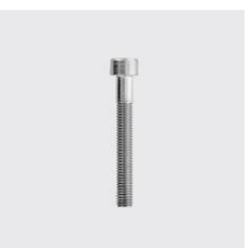
DIN 912 Vis à tête cylindrique à six pans creux, par-tiellement fileté DIN 912 Longueur mm: 45, ID unique: D912-4x45, Matériau: A2, Type de matériau: acier inoxydable, Filetage: M4, SKU 5140204045
