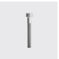
DIN 912 Vis à tête cylindrique à six pans creux, par-tiellement fileté DIN 912 Matériau: A2, Filetage: M12, Type de matériau: acier inoxydable, Longueur mm: 100, ID unique: D912-12x100, SKU 5140212100
