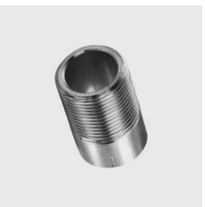
R-208-Z Anschweissnippel, Gewinde zylindrisch Materialart: Edelstahl rostbeständig, Gewinde ZOLL: 1 1/4, Unique-Id: R208-Z 1 1/4, Werkstoff: 1.4404, Länge Total mm: 35, SKU 17143545
