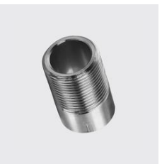
R-208-Z Anschweissnippel, Gewinde zylindrisch Materialart: Edelstahl rostbeständig, Länge Total mm: 30, Werkstoff: 1.4404, Gewinde ZOLL: 1/2, Unique-Id: R208-Z 1/2, SKU 17143530
