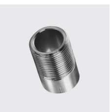
R-208-Z Anschweissnippel, Gewinde zylindrisch Gewinde ZOLL: 2, Materialart: Edelstahl rostbeständig, Unique-Id: R208-Z 2, Werkstoff: 1.4404, Länge Total mm: 40, SKU 17143555
