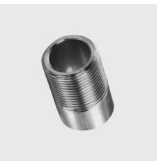
R-208-Z Anschweissnippel, Gewinde zylindrisch Materialart: Edelstahl rostbeständig, Gewinde ZOLL: 1 1/2, Werkstoff: 1.4404, Unique-Id: R208-Z 1 1/2, Länge Total mm: 35, SKU 17143550
