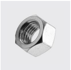
K-240 Sechskantmutter mit UNC-Gewinde Gewinde: 5/8, Materialart: Edelstahl rostbeständig, Werkstoff: A4, Unique-Id: K240+5/8, SKU 5218450
