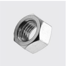
K-240 Sechskantmutter mit UNC-Gewinde Unique-Id: K240+1/2, Materialart: Edelstahl rost- beständig, Werkstoff: A4, Gewinde: 1/2, SKU 5218440
